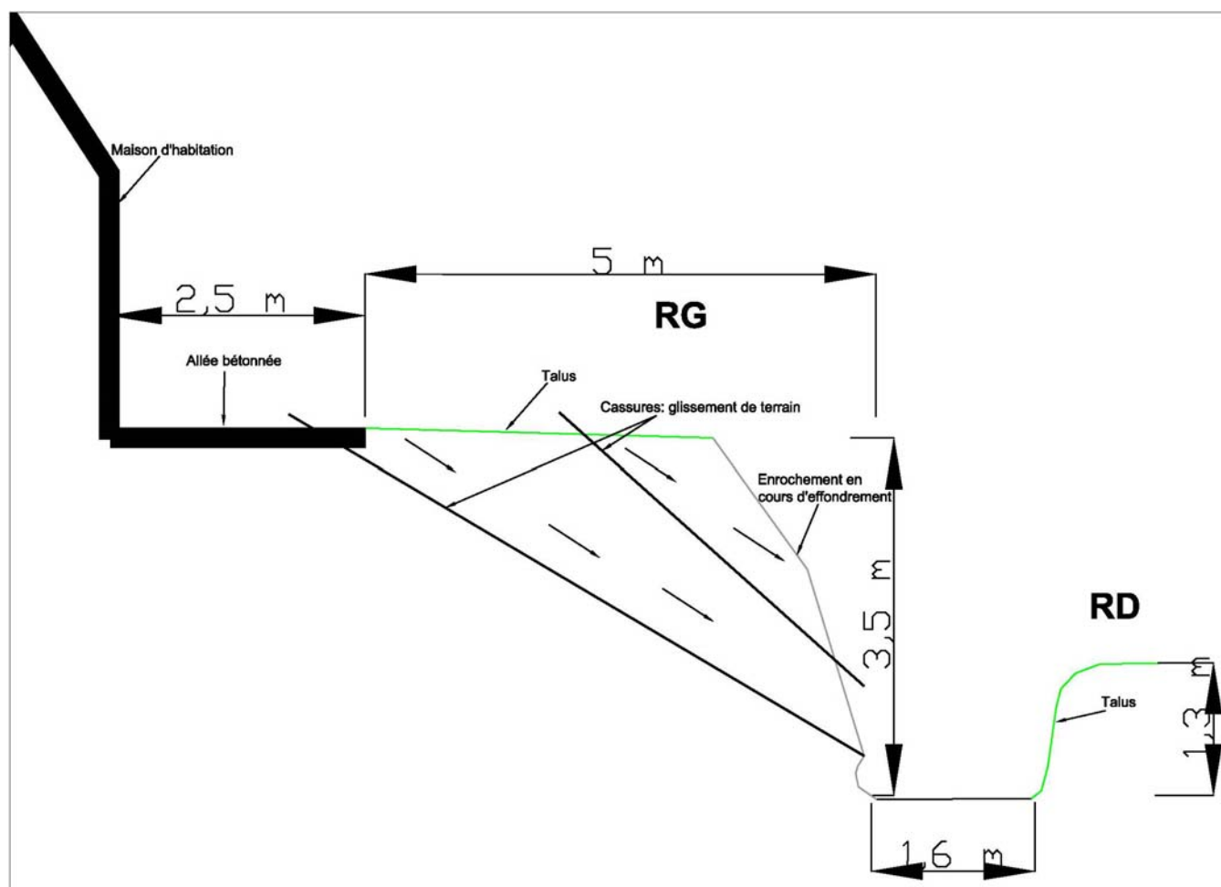
Figure 2: Schéma de l'existant – 11 rue de Fontenille
