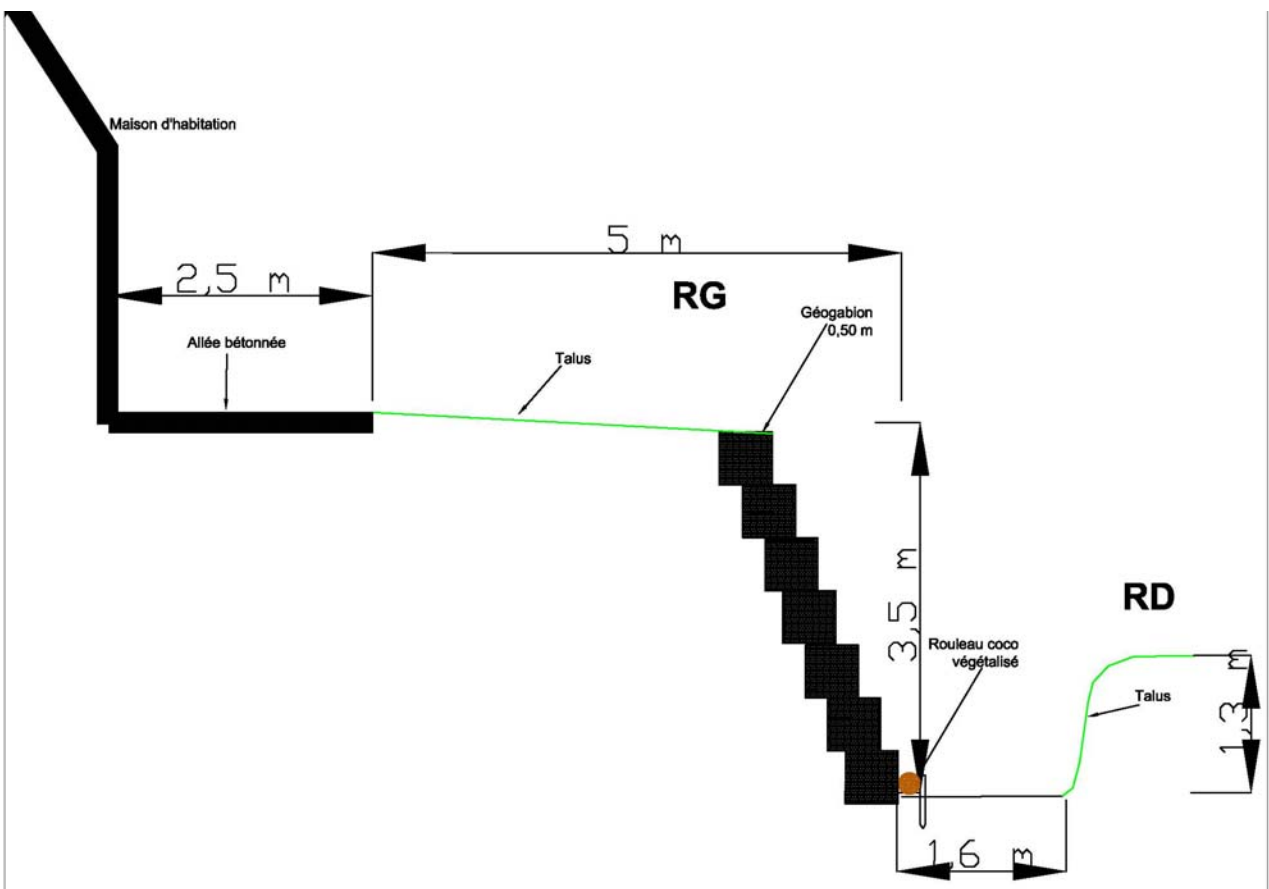
Figure 4 : Solution n°2 : Schéma de la solution proposée avec des gabions de 0,5 x 0,5 m
