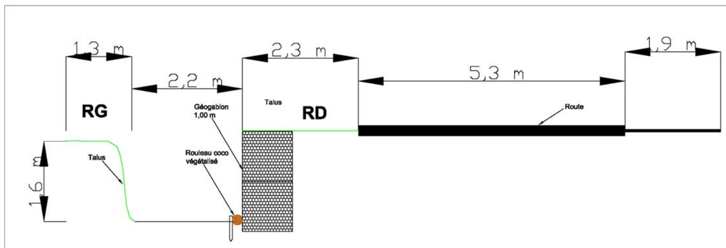
Figure 6 : Schéma d'un aménagement avec gabions de 1 m de côté et géorouleaux végétalisés
