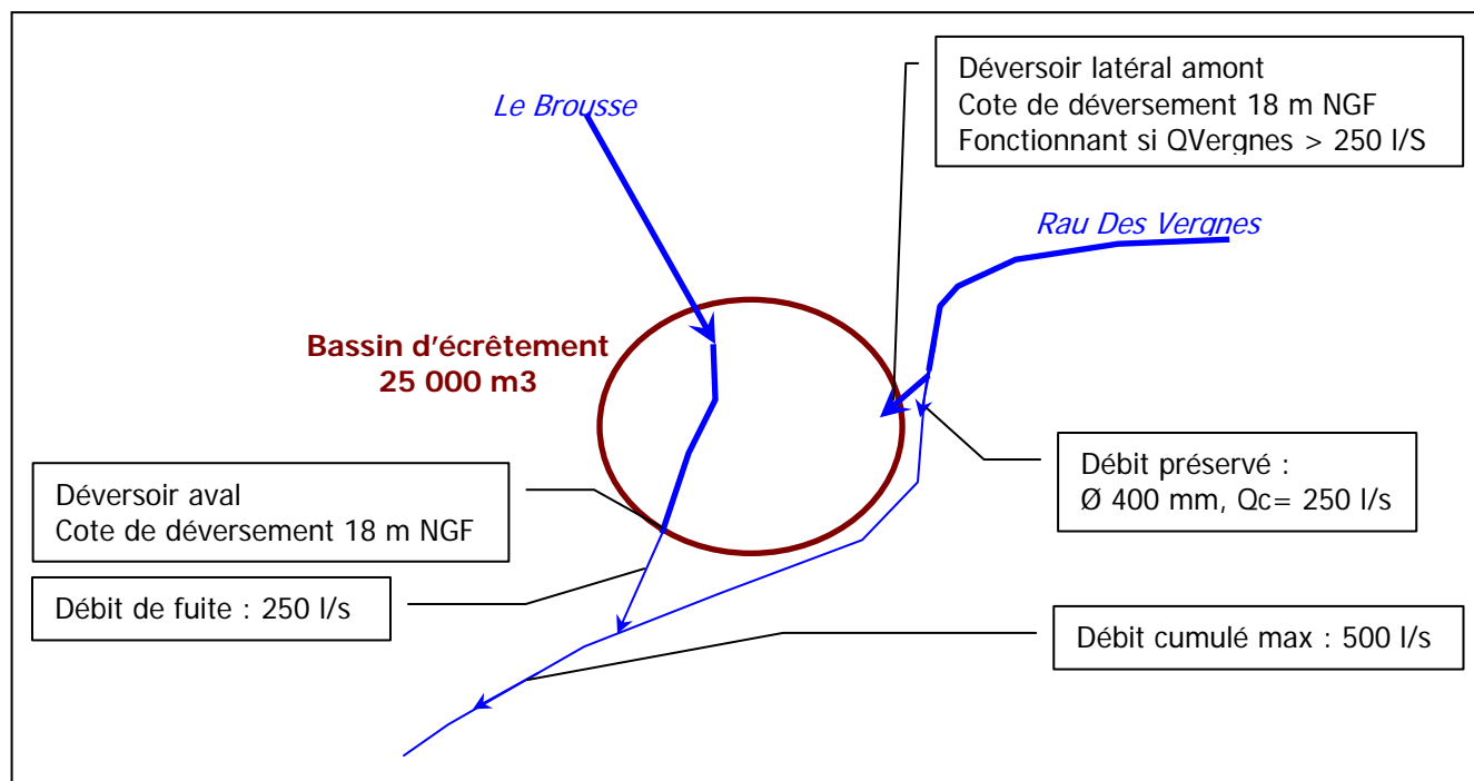
Figure 1: Schéma de principe du bassin d'écrêtement des crues
