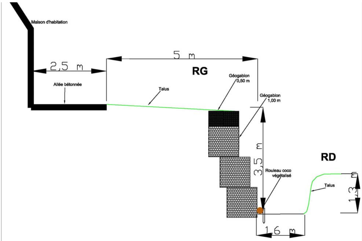
Figure 3 : Solution n°1 : Schéma de la solution proposée avec des gabions de 1 x 1 m
