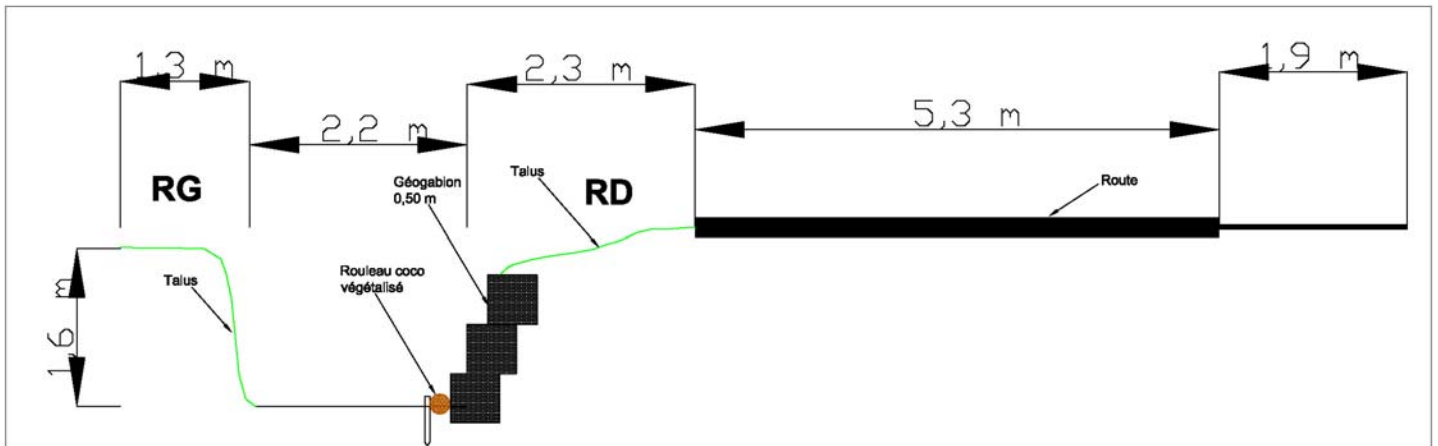
Figure 7: Schéma d'un aménagement avec gabions de 0,5 m de côté et géorouleaux végétalisés
