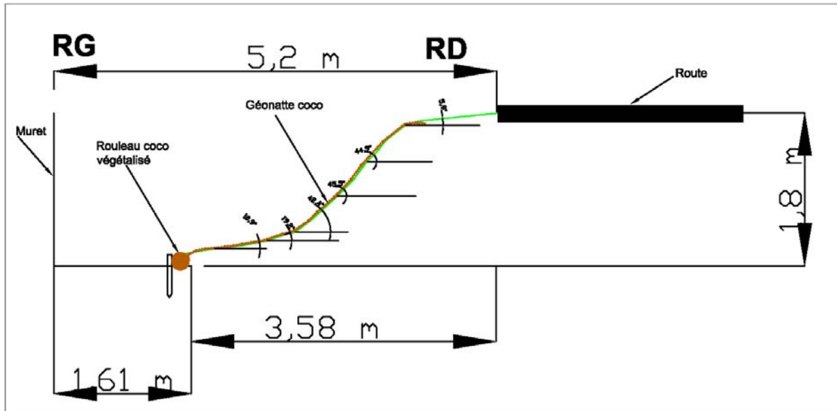
Figure 9 : Schéma du retalutage et des protections végétales
