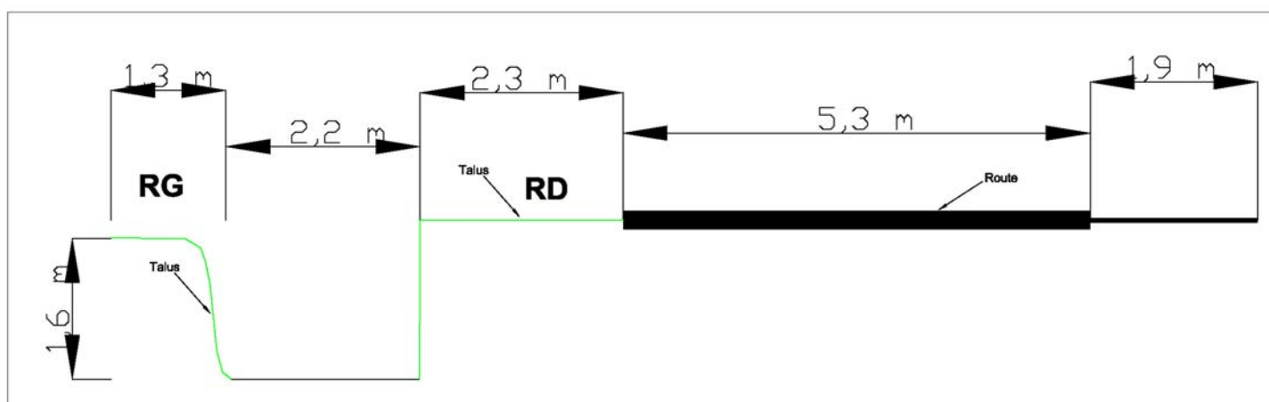
Figure 5: Schéma d'un profil transversal – Rive droite verticale -
