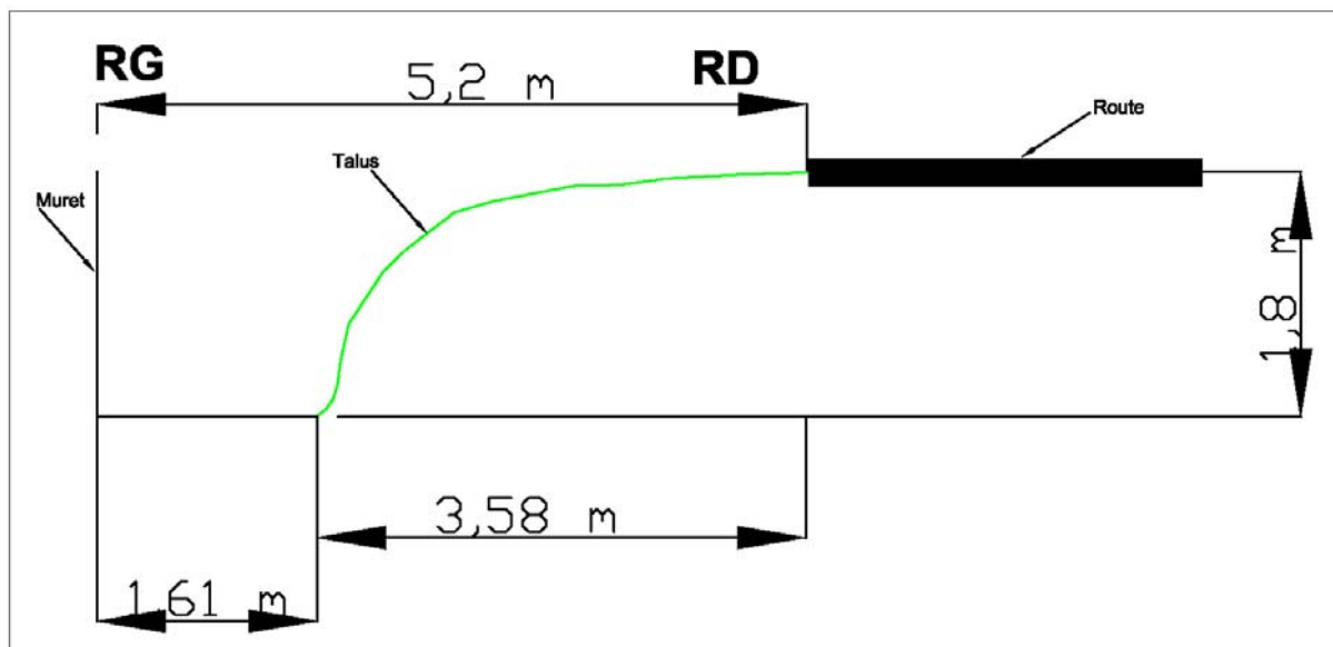
Figure 8 : Schéma d'un profil transversal – Rive droite en pente raide -Schéma d'un profil transversal – Rive droite en pente raide -
